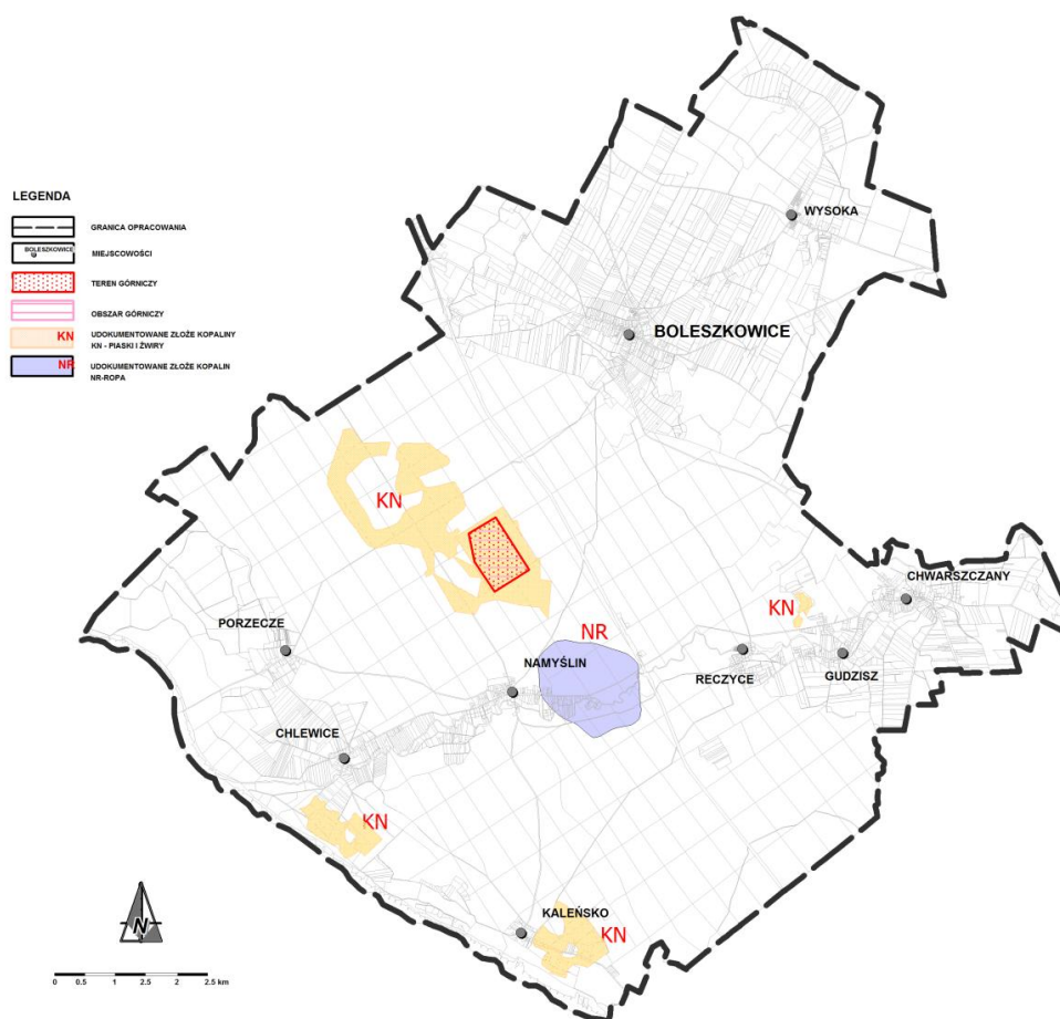
Ryc. 12 Rejony lokalizacji złóż kopalin [Źródło: opracowanie własne]
