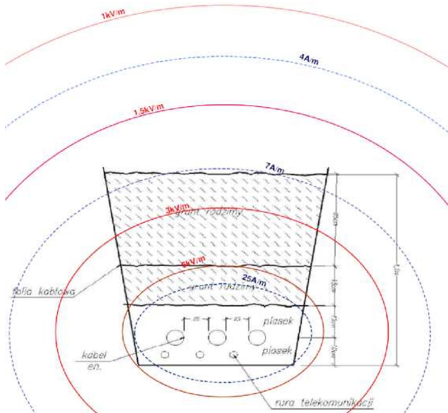
Rysunek 35. Rozkład pola elektromagnetycznego nad przykładową linią kablową średniego napięcia SN (kolorem czerwonym oznaczono izolinie pola elektrycznego, kolorem niebieskim - izolinie pola magnetycznego).
