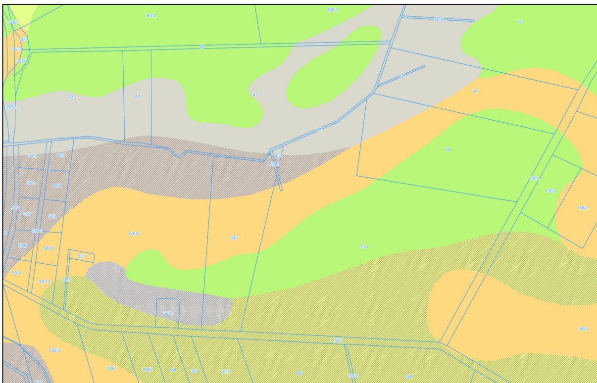
Rysunek 21. Pokrywa geologiczna obszaru inwestycji.
