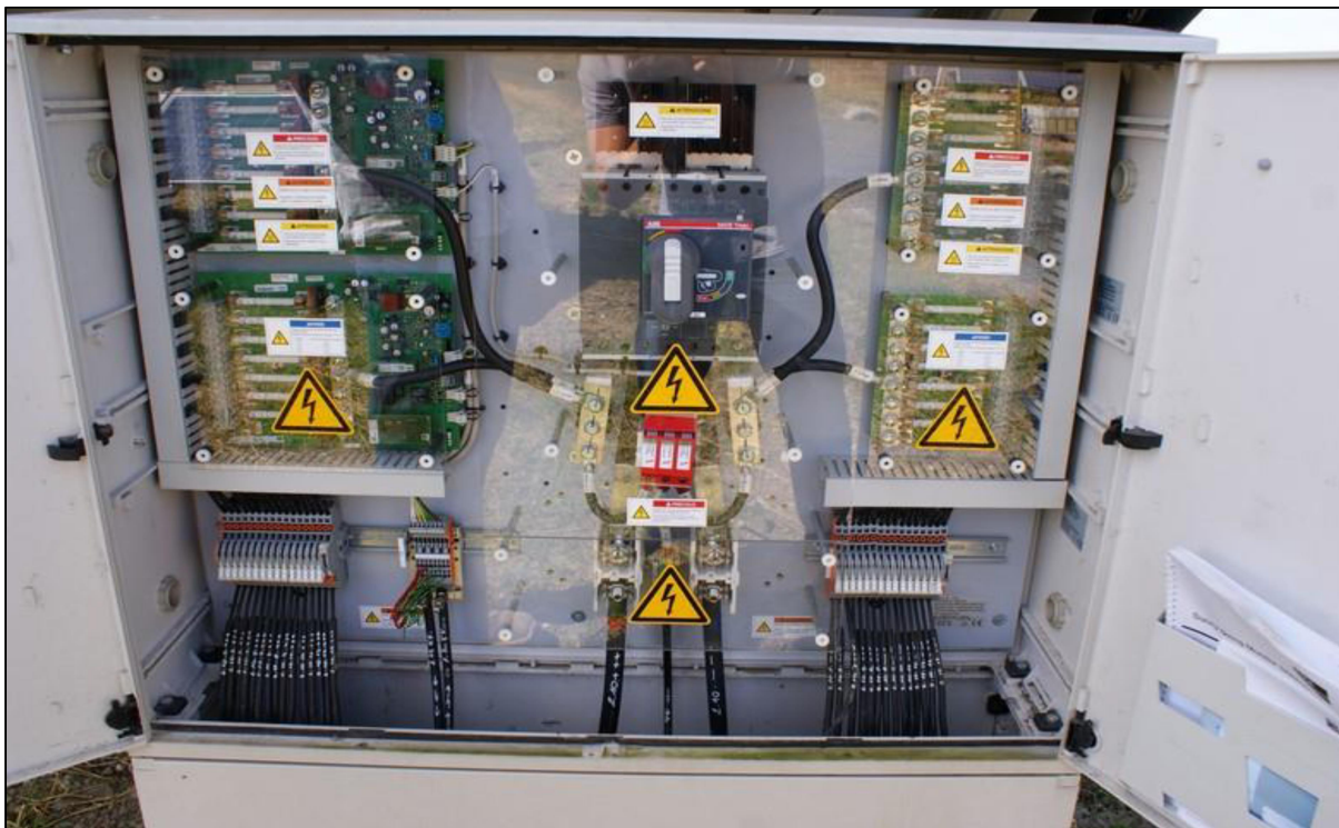
Rysunek 14. Przykład wnętrza string-box'a.
