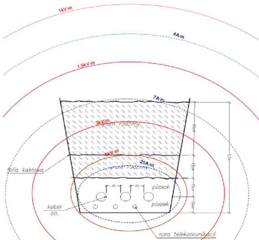
Rysunek 35. Rozkład pola elektromagnetycznego nad przykładową linią kablową średniego napięcia SN (kolorem czerwonym oznaczono izolnie pola elektrycznego, kolorem niebieskim - izolnie pola magnetycznego).
