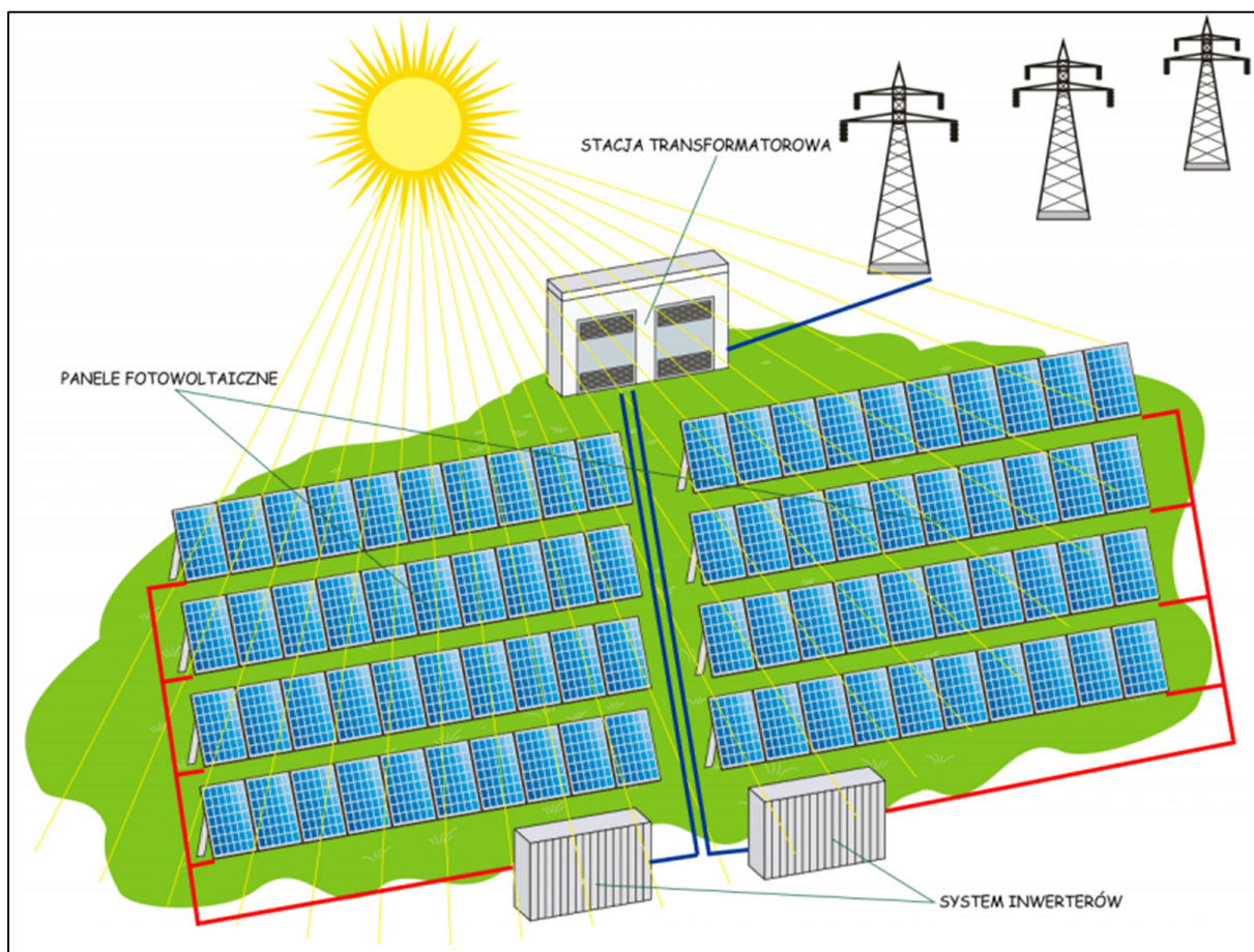
Rysunek 10. Uproszczony proces działania elektrowni fotowoltaicznej (źródło: Photonlab Systemy Fotowoltaiczne AIP Jakub Wiśniewski, Politechnika Warszawska)
