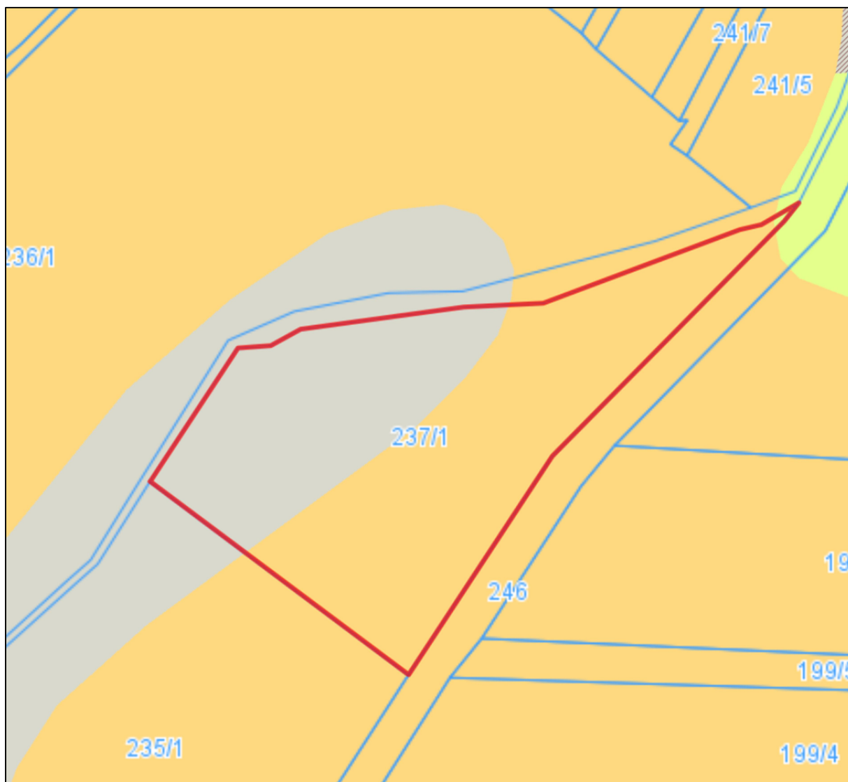
Rysunek 19. Pokrywa geologiczna obszaru inwestycji.
